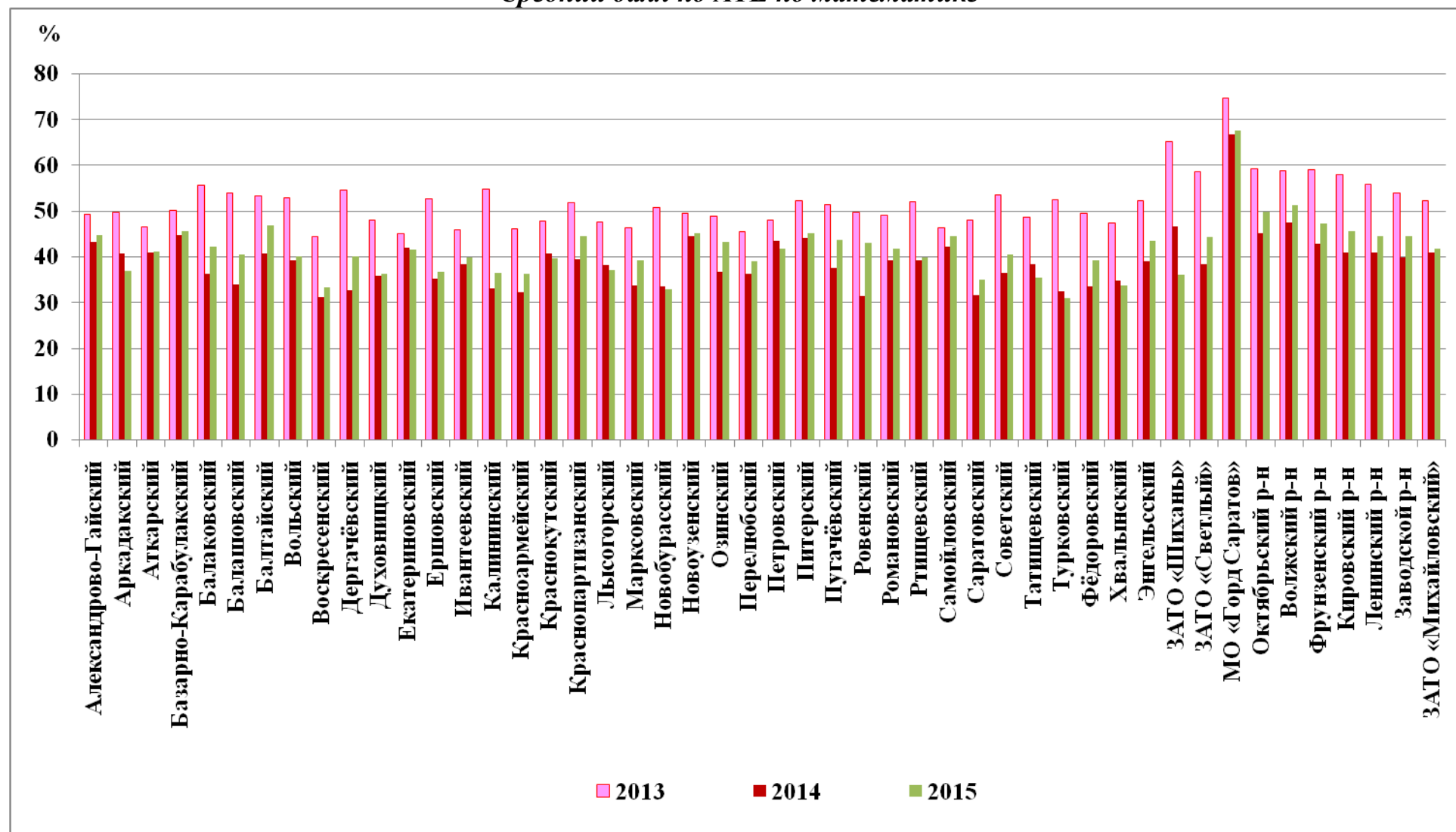
Средний балл по АТЕ по математике
