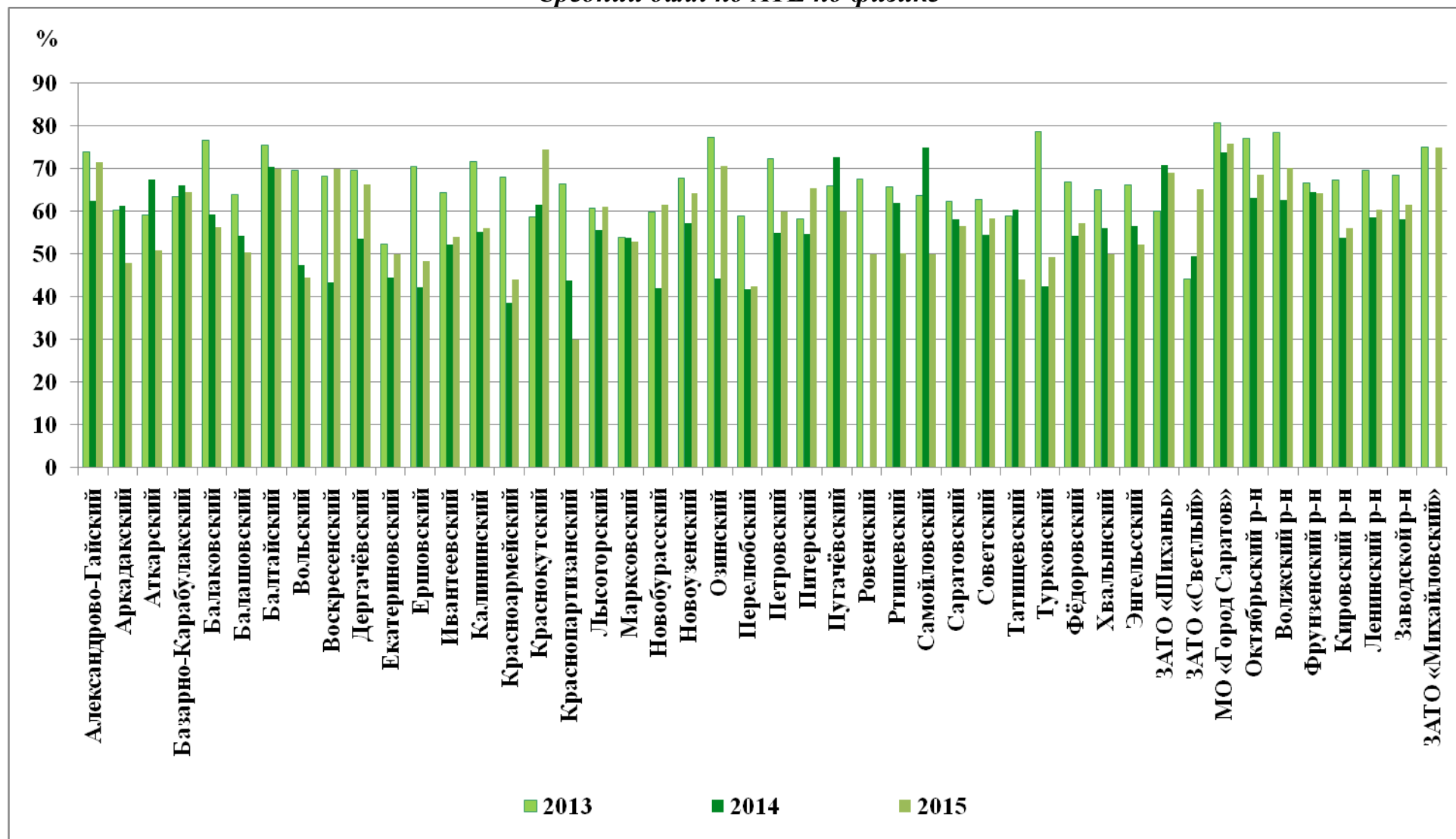
Средний балл по АТЕ по физике
